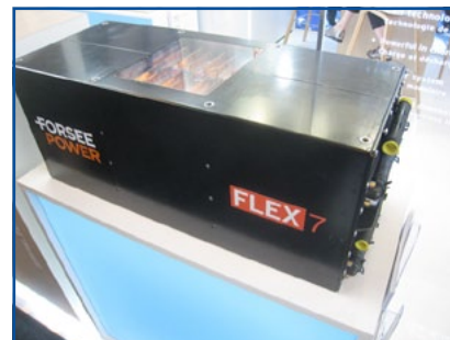
FORSEE POWER - Pacchi batterie NMC da 7 a 35 kWh collegabili in serie o parallelo.
