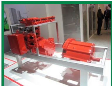
CUMMINS - Sistema di elettrificazione a batterie o in combinazione con un compatto motogeneratore.
